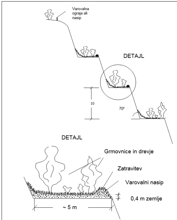
Slika 8: Rekultivacija etažnih ravnin
